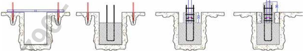
Şekil 1. Ankraj Çukuru ve Betonunu Kesiti
